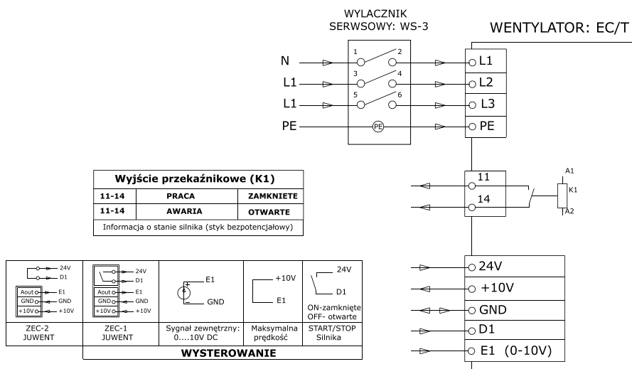
Rys. 2 Schemat podłączenia i sterowania wentylatora: WDV-EC/T-[-35, -40, -45, -50, -56,]
