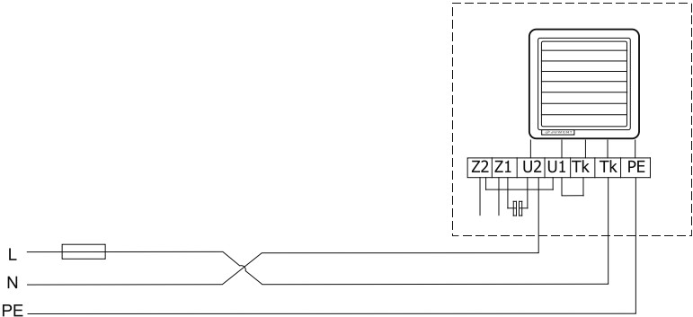
Rys. 2. Schemat połączeń elektrycznych bez automatyki.
