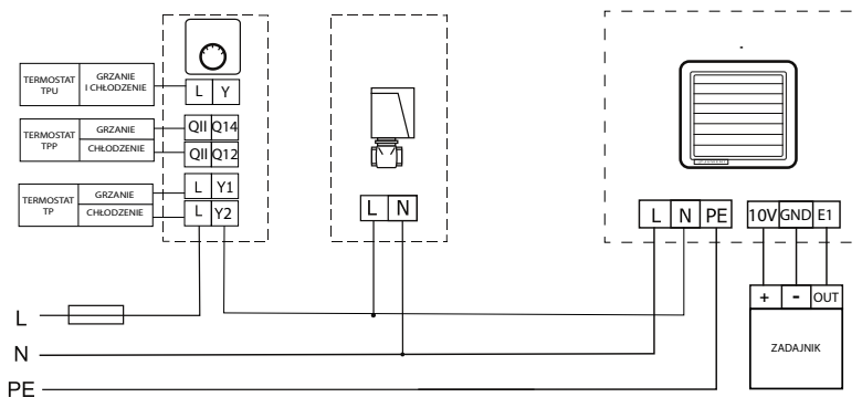
Rys. 8. Schemat połączeń elektrycznych z automatyką (termostat steruje, siłownikiem zaworu i pracą wentylatora)
