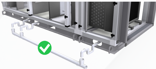
Poprawne wykonanie instalacji odprowadzenia skroplin.
