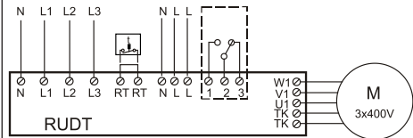
Fig. 16 RUDT controller
