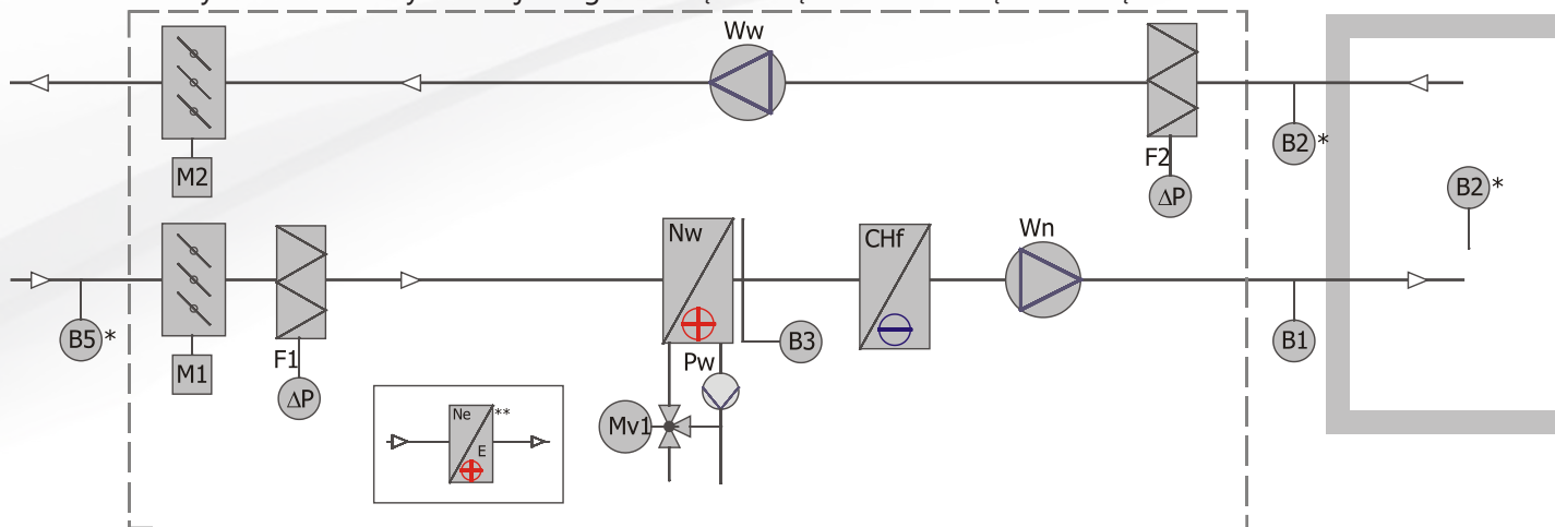
Układ automatyki nawiewno-wywiewnej z nagrzewnicą wodną oraz chłodnicą freonową
