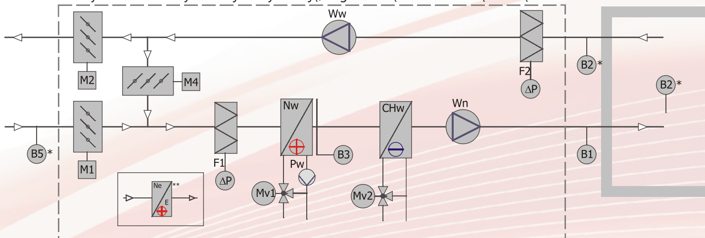
Układ automatyki nawiewno-wywiewnej z recyrkulacją, nagrzewnicą oraz chłodnicą wodną
