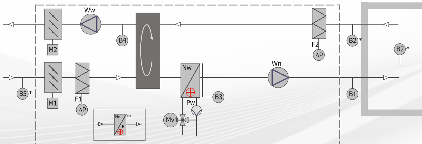
Układ automatyki nawiewno-wywiewnej z wymiennikiem obrotowym, nagrzewnicą i chłodnicą wodną
