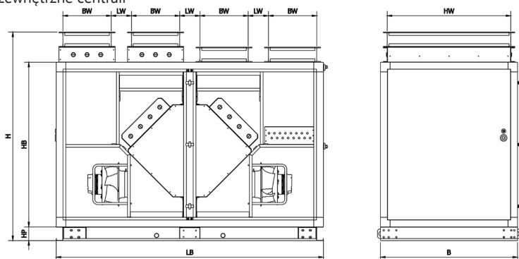
Rys.4. Wymiary zewnętrzne centrali
