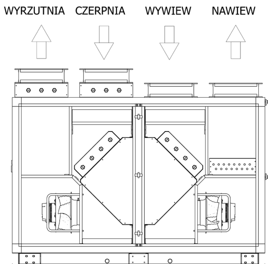
Rys.2. Strona obsługi prawa.
