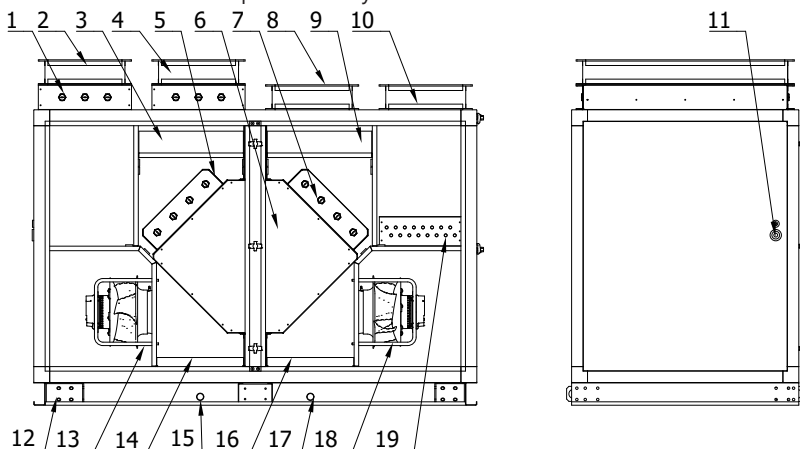
Rys.1. Przykładowa konfiguracja centrali.
