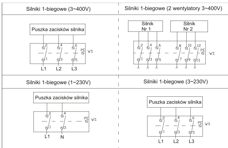
Rys.6. Schematy połączeń wyłącznika serwisowego WS z silnikiem jedno lub trójfazowym
