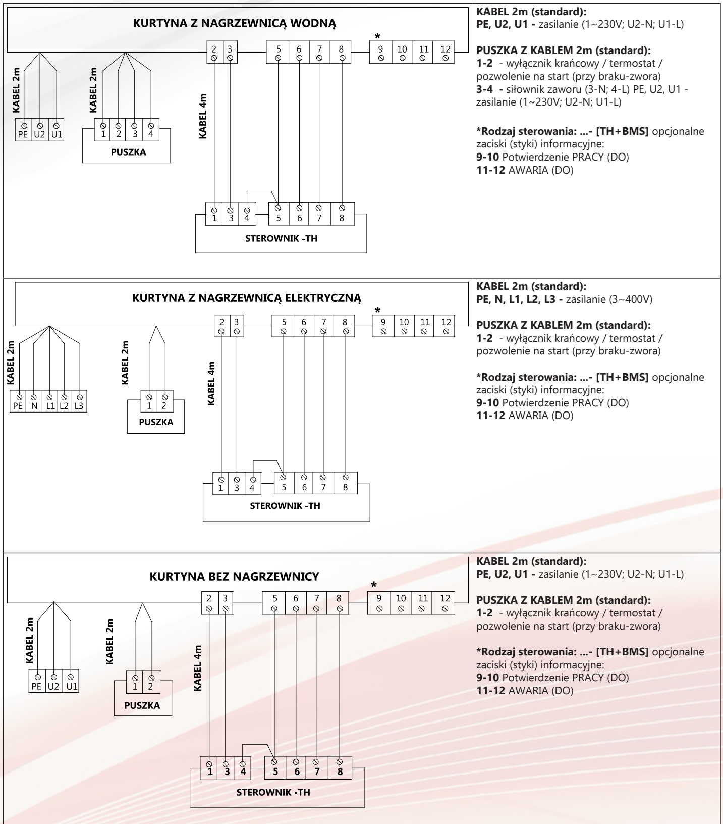
Rys. 63. Schemat blokowy podłączenia kurtyń: SILVER/GOLD/SMART-...-[-W;-Z;-E] z sterownikiem [TH] oraz sterownikiem TH z BMS sterowanie [TH+BMS]
