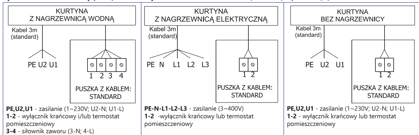
Rys. 59. Schemat blokowy podłączenia kurtyln: SILVER/GOLD/SMART-...[-W;-Z;-E] z pilotem [A]
