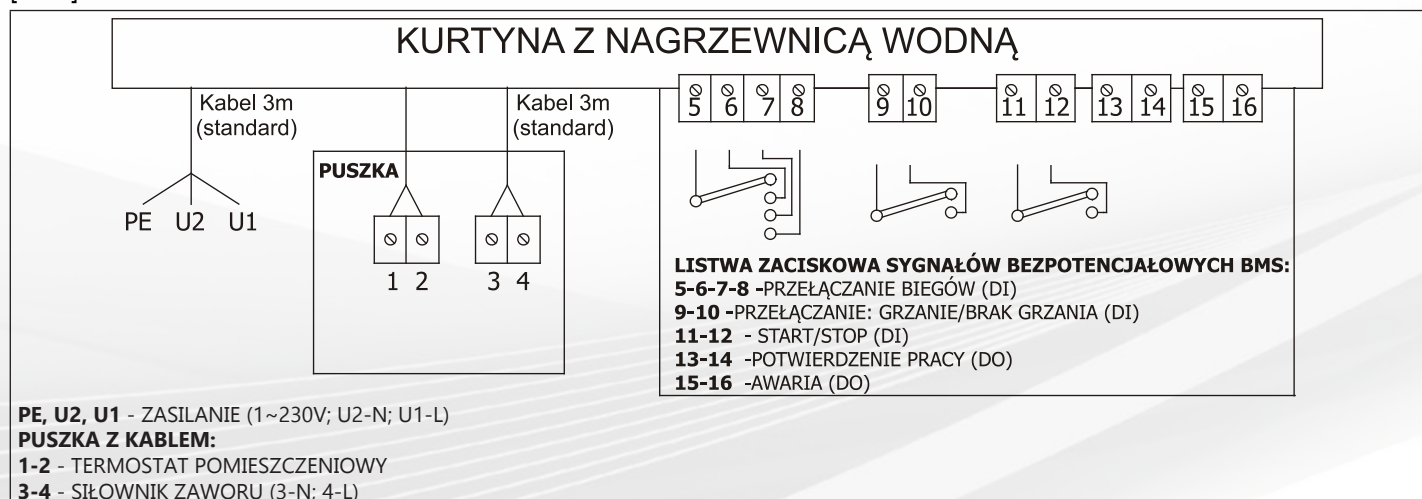
Rys. 62. Schemat blokowy podłączenia kurtyń: SILVER/GOLD/SMART-...[-W;-Z;-E] bez pilota z dodatkowym sterowaniem [BMS]
