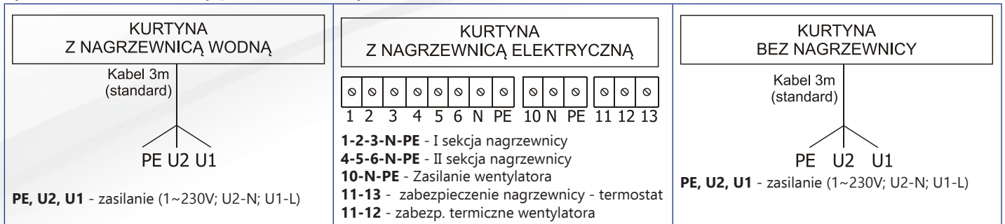
Rys. 60. Schemat blokowy podłączenia kurtyń: SILVER/GOLD/SMART-...-[-W;-Z;-E] bez sterowania [B]
