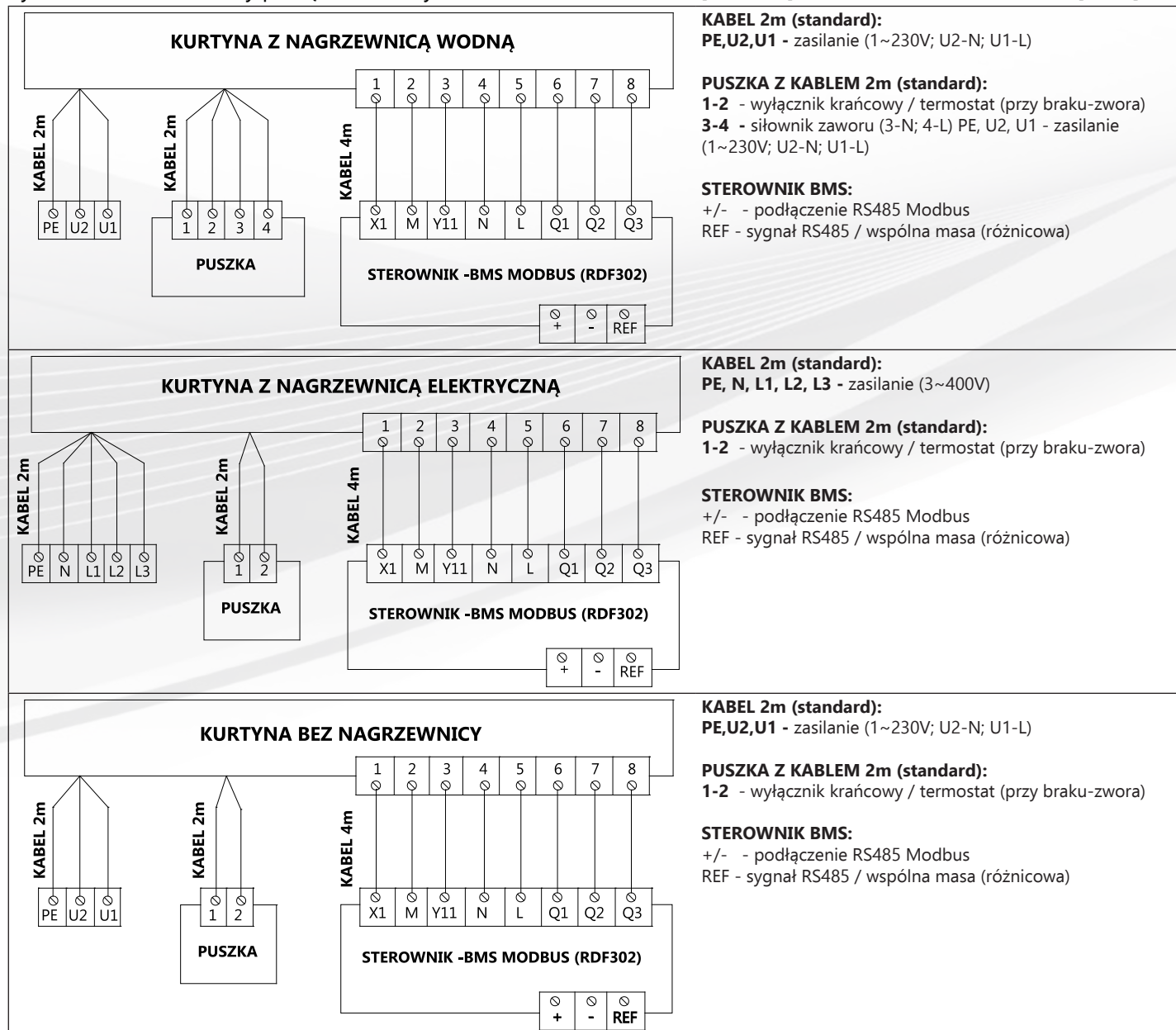
Rys. 64. Schemat blokowy podłączenia kurtyny: SILVER/GOLD/SMART-...[-W;-Z;-E] z sterowaniem BMS Modbus[MOB]
