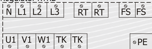
Rys. 55. Regulator RTRD
