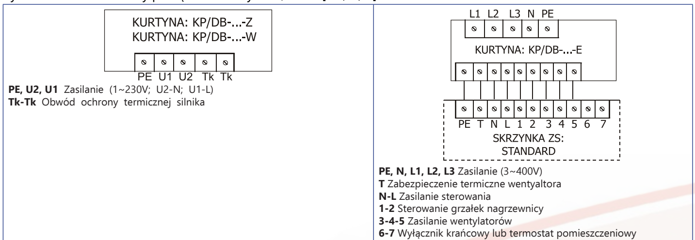
Rys. 67. Schemat blokowy podłączenia kurtyń: KP/BB-...-[-W;-Z;-]-[-J;-T], KP/BB ECONOMIC-...-W-[-J;-T] oraz KP/BN-...-[-W;-Z;-]-[-J;-T]
