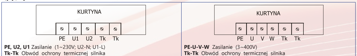
Rys. 68. Schemat blokowy podłączenia kurtyń: KP/BB-...-E-T
