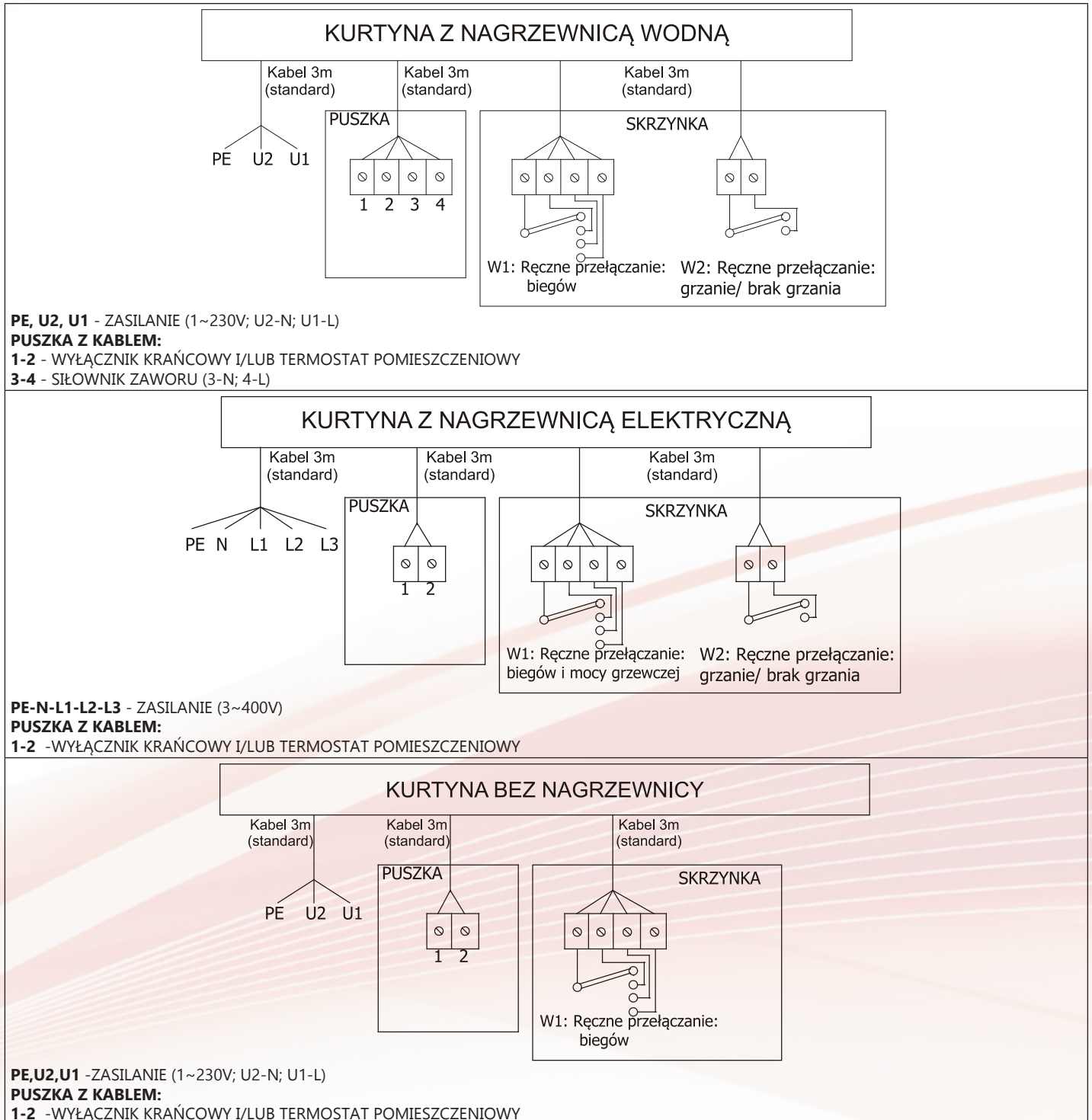
Rys. 61. Schemat blokowy podłączenia kurtyń: SILVER/GOLD/SMART-...-[-W;-Z;-E] ze skrzynką[S]
