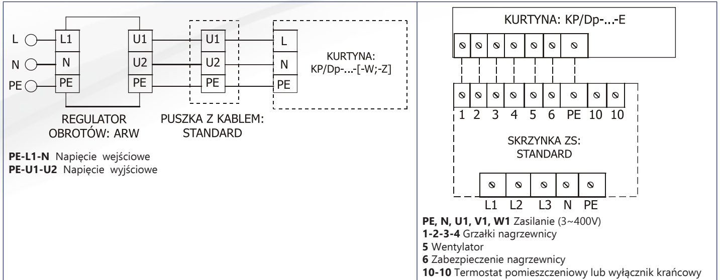
Rys. 66. Schemat blokowy podłączenia kurtyń: KP/DB-...-[-W;-Z;-E]
