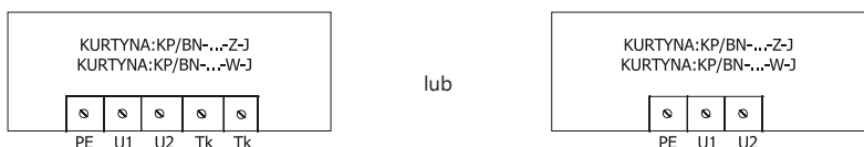
Rys. 1 Schemat blokowy podłączenia kurtyń: KP/BN-...-[-W;-Z;-]J
